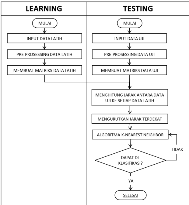
Gambar 2.3 Tahapan proses klasifikasi dengan KNN
