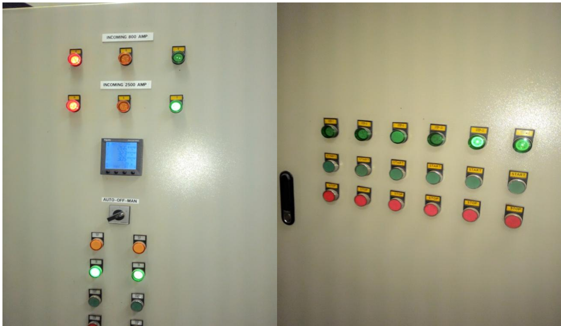
Gambar : Bagian Luar Panel Capasitor Bank di Gedung Power House PLT Biomassa Bantar Gebang
