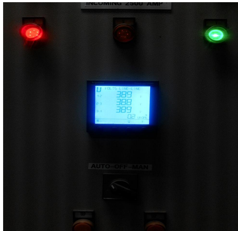
Gambar : Pengukuran Arus dan Tegangan pada Panel LVMDB Auxiliary
