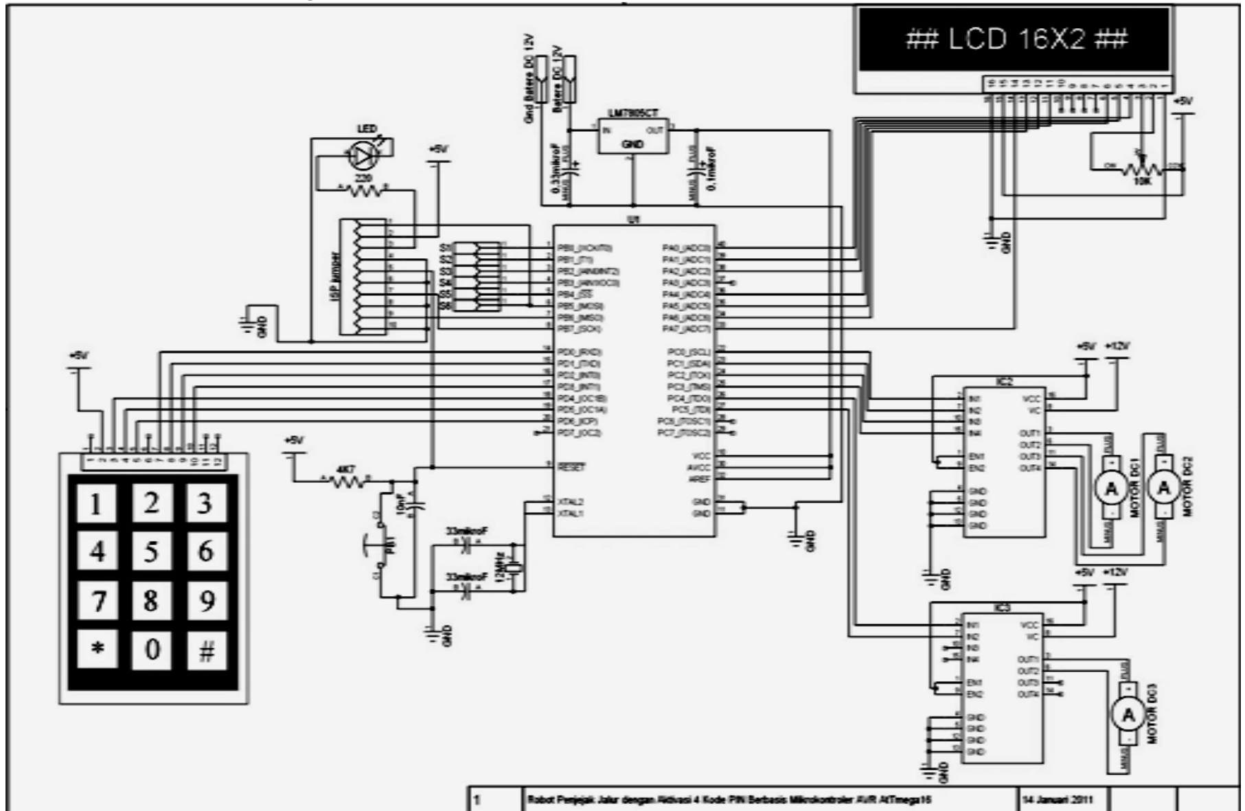
Lampiran 5: Skema Rangkaian Keseluruhan Alat Robot Penjejak Jalur Dengan Sistem Aktivasi 4 Kode PIN Berbasis Mikrokontroler AVR ATmega16
