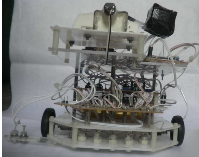
a. Robot Tampak Depan
