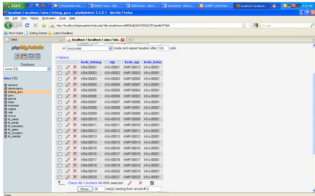
Gambar 4.16 Database bidang_guru
