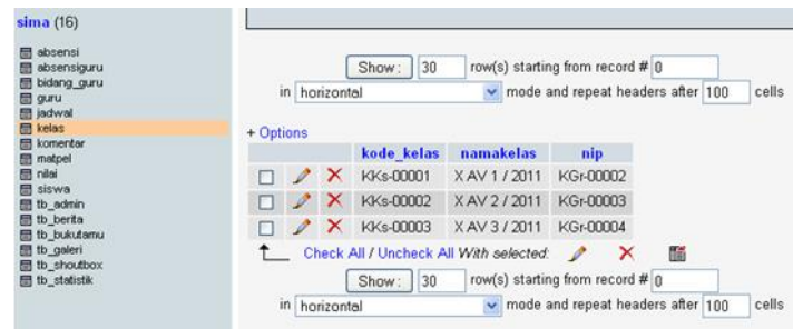
Gambar 4.18 Database kelas
