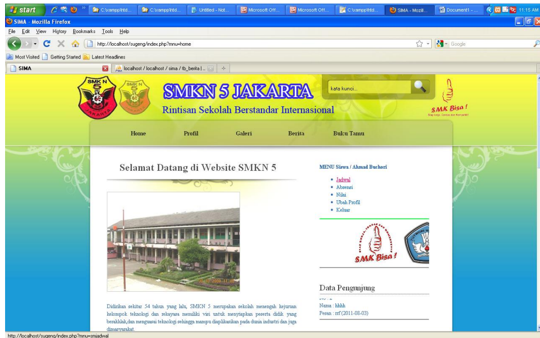
Gambar 4.33 Halaman siswa
